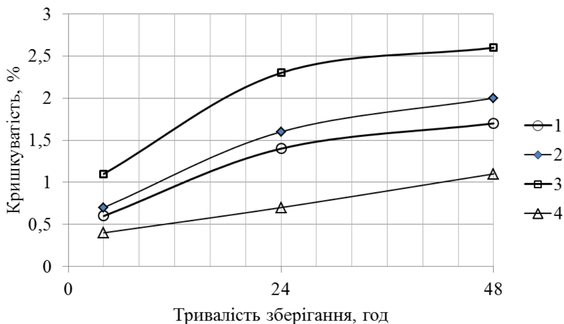
Рис. 2. Кришкуватість м'якушки безглютенового хліба, %:
