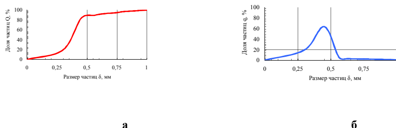
Рис. 1. Интегральная (а) и дифференциальная (б) кривые распределения частиц по размерам
