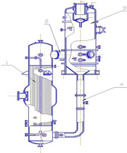
Рис. 1. Випарний апарат
