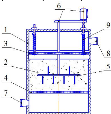
Рис.1. Адсорбер для зневоднення етанолу: 1 – корпус; 2 – сорбуючий шар (адсорбент); 3, 4 – обмежувальні решітки; 5 – розпушувач сорбенту; 6 – привід розпушувача; 7, 8 – патрубки; 9 – притиски
