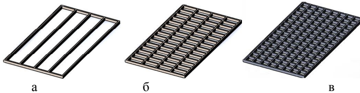
Рис.1. Конструкції ріжучо-перемішуючих пристроїв: а – з вертикальними пластинами, б – з комітками прямокутної форми, в – з комітками квадратної форми
