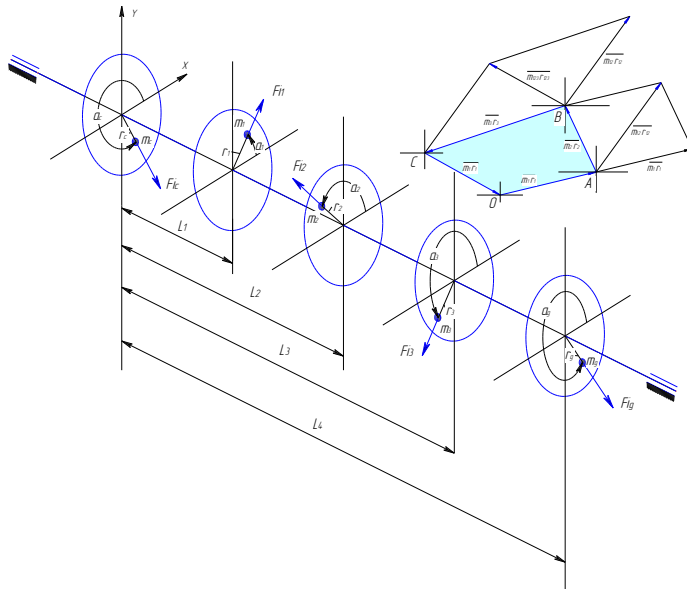
Рис. 1. Схема до визначення параметрів зрівноваження ротора
