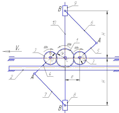
Рис. 1. Схема механізму привода вузла поперечного зварювання плівки: 1 – приводне зубчасте колесо; 2 – нерухома зубчата рейка; 3, 4, 5 – ведені зубчасті колеса; 6, 7 – шатуни; 8, 9 – зварні елементи; 10 – рама; 11 – конвеєрна стрічка.
