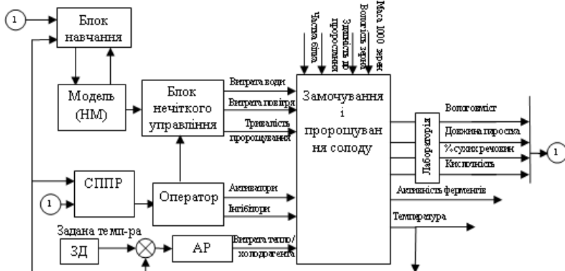
Рис. 1. Інтелектуальна система управління замочуванням і пророщуванням солоду.
