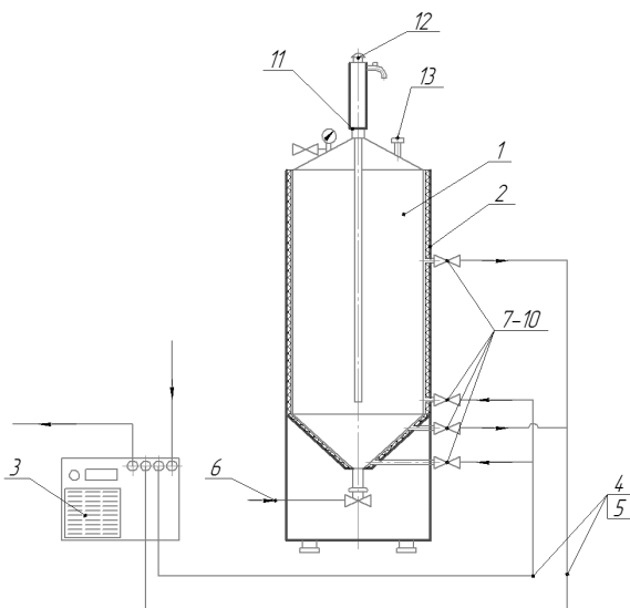
Рис.1. Доброджувальна установка
