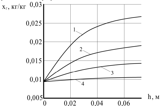
Зміна вологовмісту повітря по висоті псевдозрідженого шару матеріалу в чотирьохсекційній сушці, де 1, 2, 3 та 4 відповідно номера секцій
