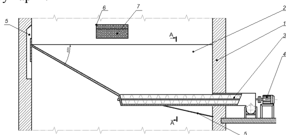
Рис. 1. Трьохярусна солодосушарка
