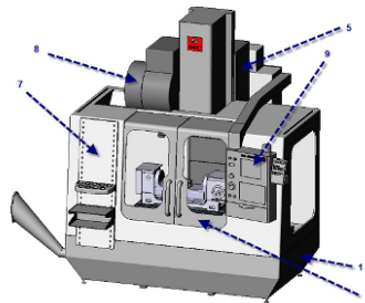
Рис. 1. Корпус вертикально-фрезерного верстата із ЧПУ
