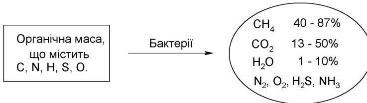
Схема переробки органічної біомаси
