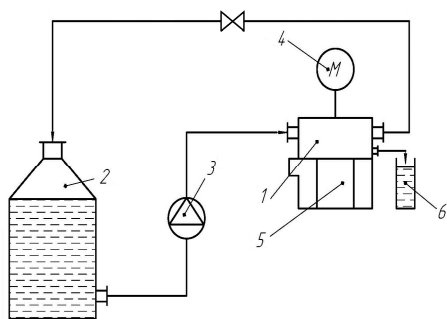
Рис. 1. Будава ультрафільтраційної установки:
