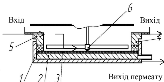
Рис. 2. Будава ультрафільтраційної комірки:
