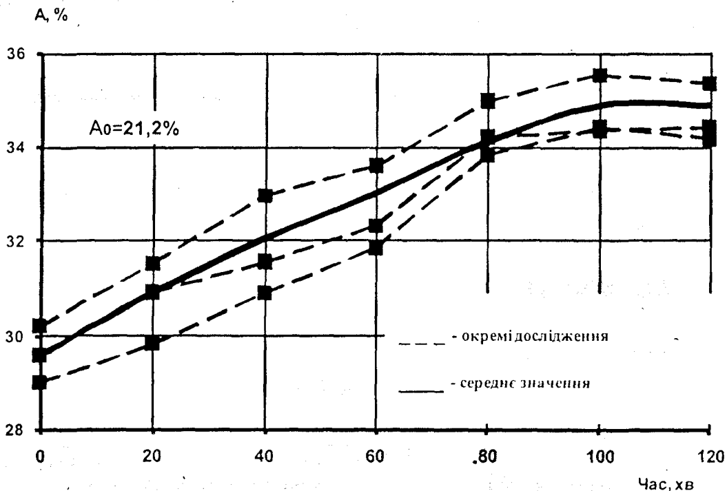
Рис. 3. Вплив тривалості витримки обробленої електрогідралічними розрядами водно-цементної суспензії на її активність (A)
