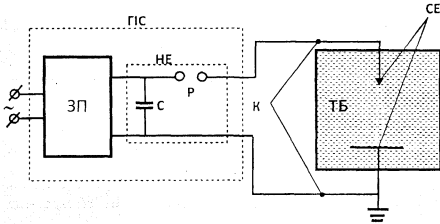
Рис. 1. Принципова електрична схема електрогідравлічної установки
