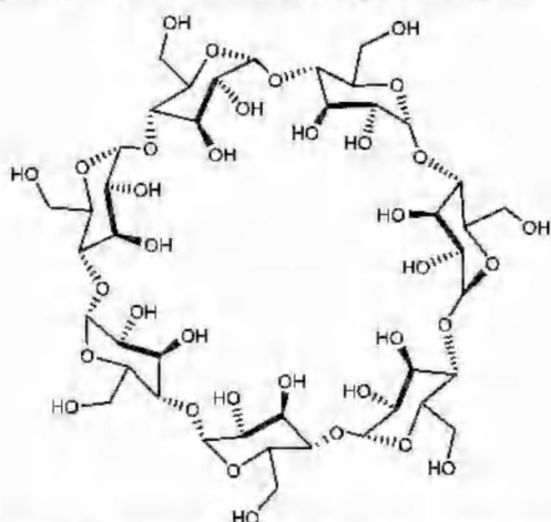
Рис. 2. Структурна формула \beta -циклодекстрину
