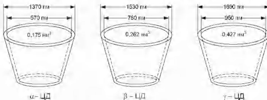
Рис. 1. Приблизний геометричний розмір і об'єм циклодекстринів
