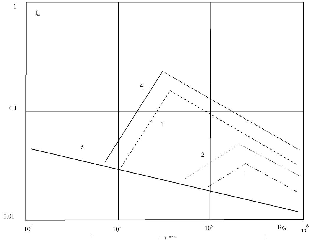
Рис.1. Залежність f_{ia} від Re_r : 1- Re_p=1000 (1); 2- Re_p=2000 (1); 3- Re_p=1000 (2); 4- Re_p=2000 (2); 5- f_{ia} = 0,182 Re_r^{-0,2} .
