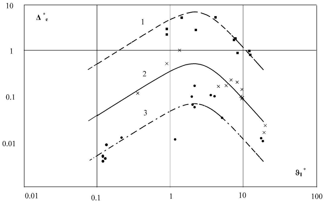
Рис. 2. Залежність \Delta_e^* = f(\theta_1^*) : Розрахунок за (7): 1- Re=950 , We=4500 ; 2- Re=600 , We=5500 ; 3- Re=300 , We=4500 . Дослідні дані \blacksquare - Re_p=800-1100 , We=4000-5000 ; \times - Re=500-700 , We=5000-6000 ; \bullet - Re=200-400 , We=4000-5000 .
