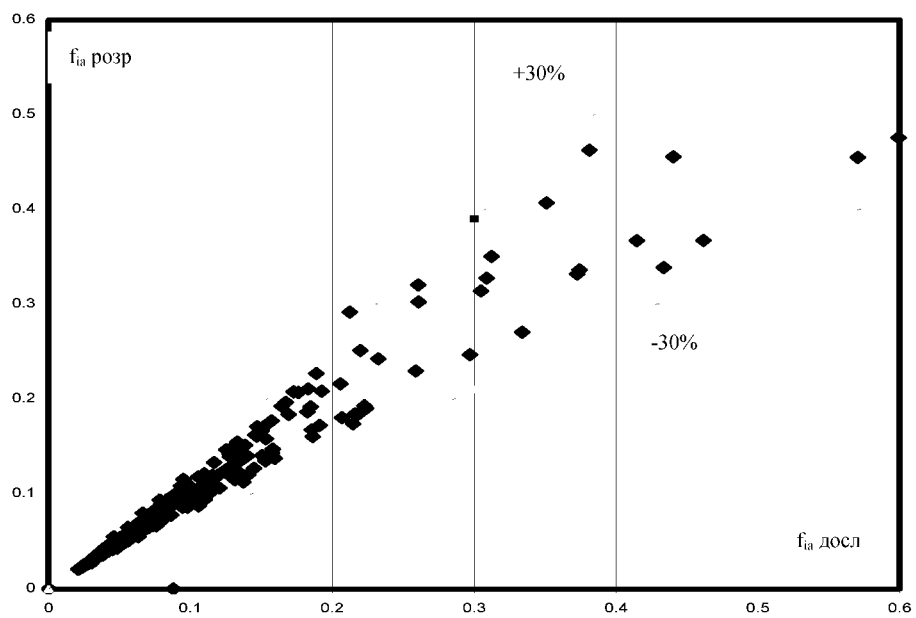
Рис.4. Порівняння розрахованих та дослідних значень f_{ia}
