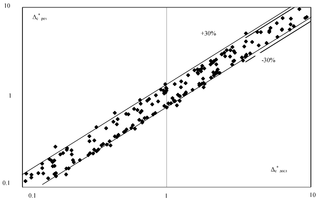
Рис.3. Порівняння розрахованих за (7) та дослідних значень \Delta_{\epsilon}^*
