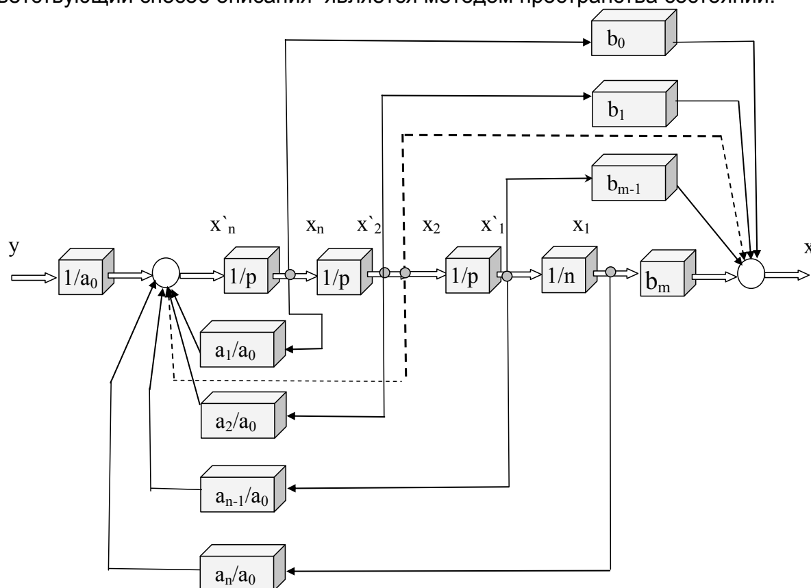
Рис. 3. Модель объекта исследования (оборудования) в переменных состояния
