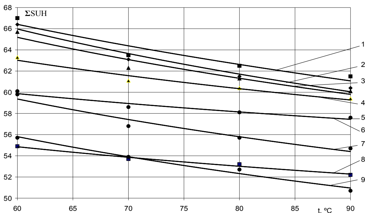
Рисунок 3. Зміна вмісту загальної кількості цукрів у плодах глоду, висушених контактним методом, %: 1 – глід Мейера; 2 – глід алма-атинський; 3 – Шаміль; 4 – глід східний; 5 – Людмил; 6 – Збігнев; 7 – Мао Мао; 8 – Китайський 1; 9 – Глід одноматочковий
