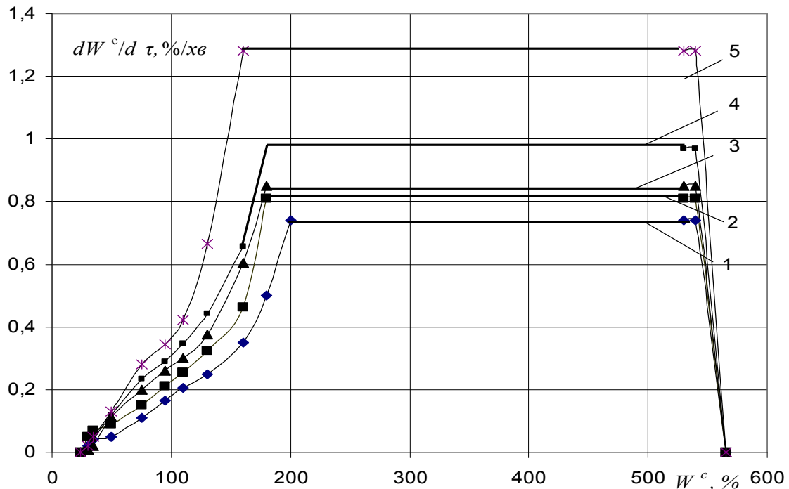
Рисунок 2. Криві швидкості контактного сушіння глоду сорту Збігнєв при температурах, °C: 1 – 60. 2 – 70. 3 – 80. 4 – 90. 5 – 100
