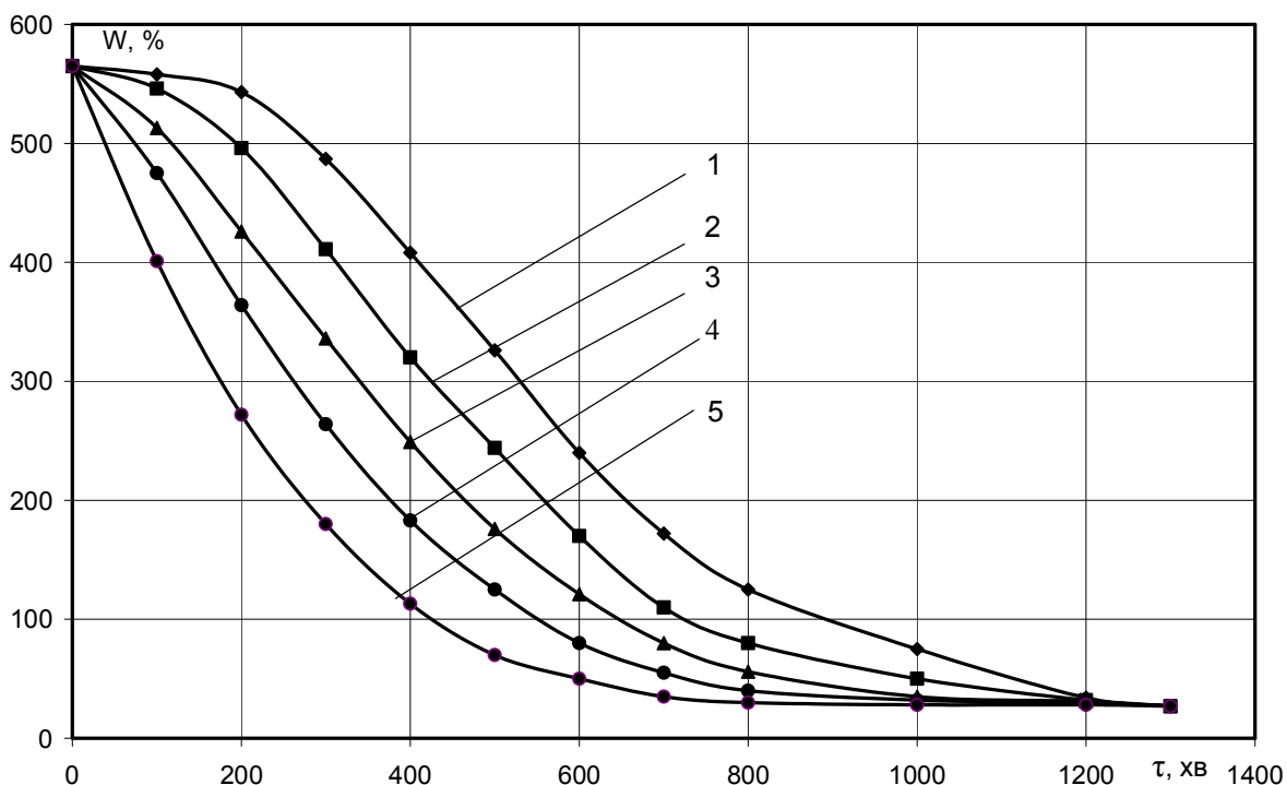
Рисунок 1. Криві контактної сушіння глуду сорту Збігнєв при температурах, 0 С: 1 – 60, 2 – 70, 3 – 80, 4 – 90, 5 – 100
