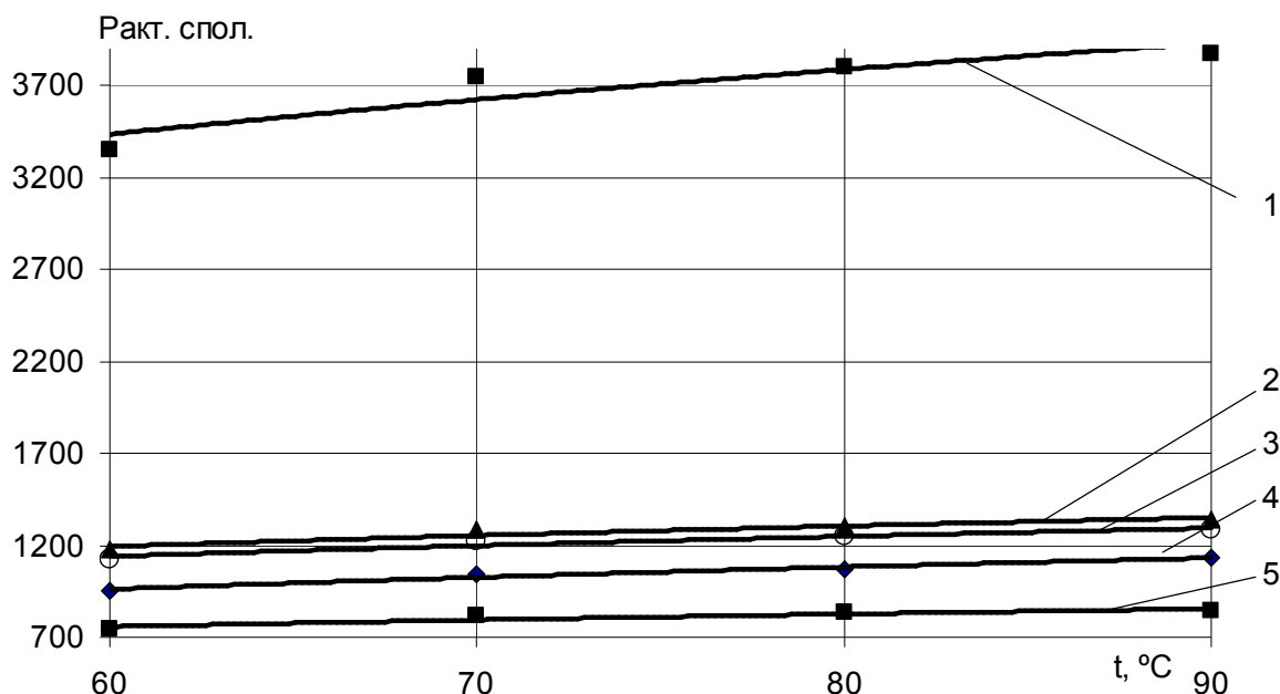
Рисунок 5. Вміст загальної кількості поліфенолів у плодах глоду висушених контактним методом, мг/100 г: 1 – глід одноматочковий; 2 – глід алма-атинський; 3 – Збігнев; 4 – Шаміль; 5 – Людмил
