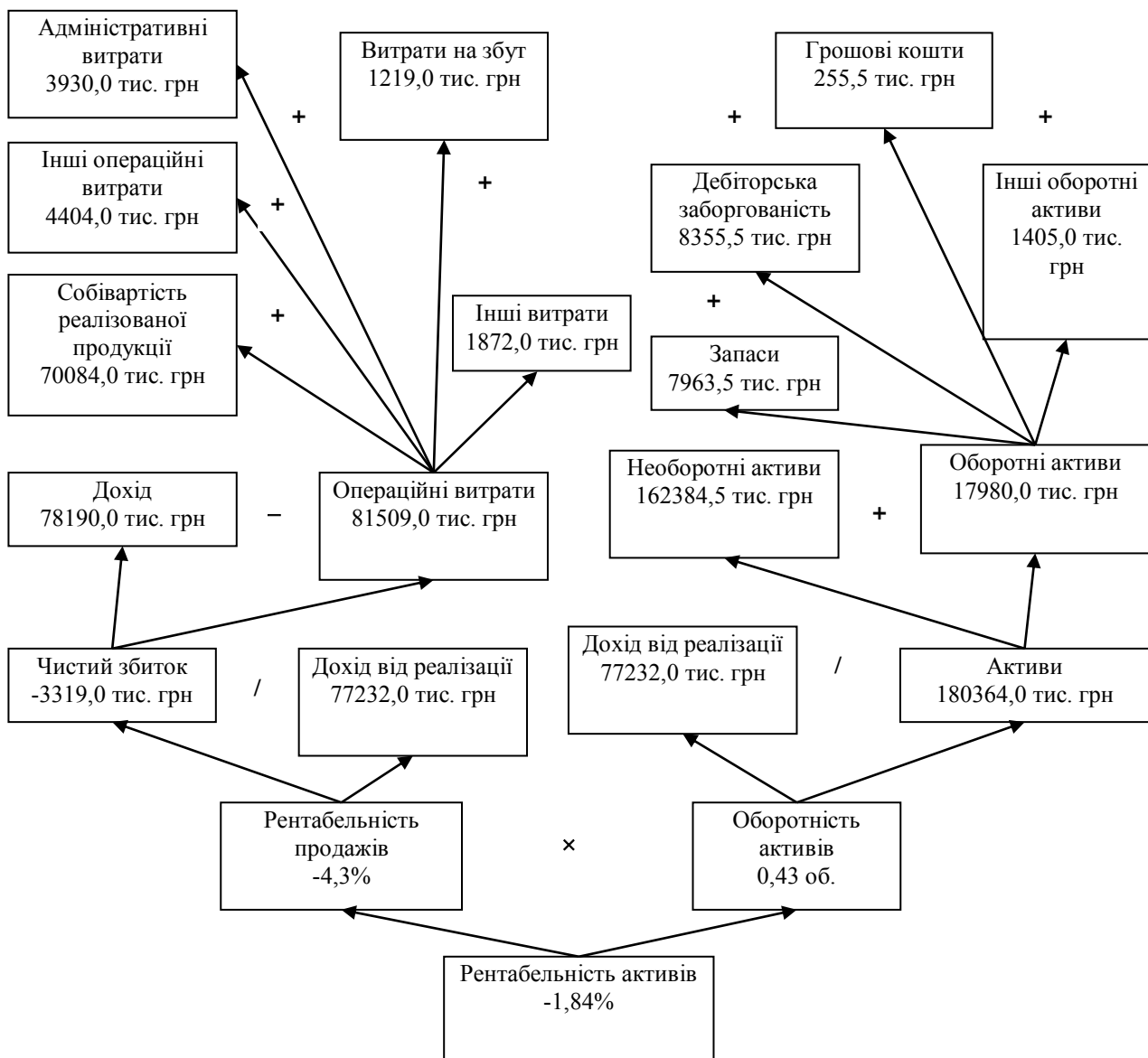
Рис. 1. Модель Дюпона для показника рентабельності сукупного капіталу ПАТ ДПЗКУ “Кролевецький комбінат хлібопродуктів” на основі даних 2018 р.
