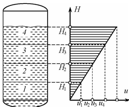
Рис. 1. Схема визначення висотного розподілу газотримувальної здатності за показником генерування \text{CO}_2
