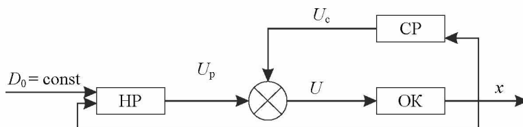
Рис. 1. Структура нечіткої АСР
