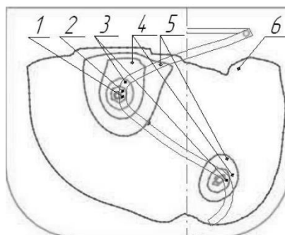
Рисунок 4 – Изолинии скорости вокруг рабочего органа машины Л4-ХТБ
