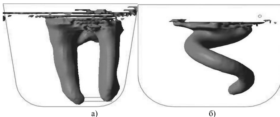
Рисунок 2 – Исоповерхности вязкости вокруг рабочего органа: а) - А2-ХТБ; б) - Л4-ХТБ
