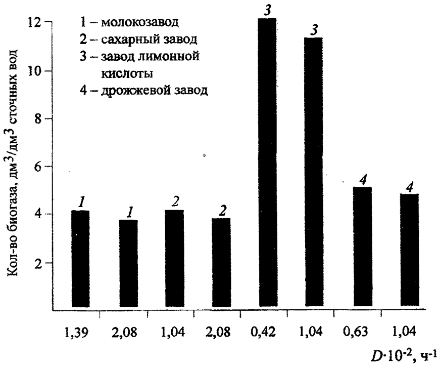
Рис. 1. Выход биогаза при очистке сточных вод предприятий пищевой промышленности в зависимости от скорости разбавления.
