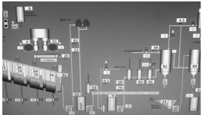
Рис.5. Мнемосхема станції нагрівання дифузійного соку
