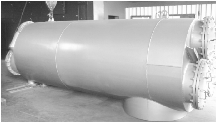
Рис.1. Підігрівник ПДСУ-1600-3
