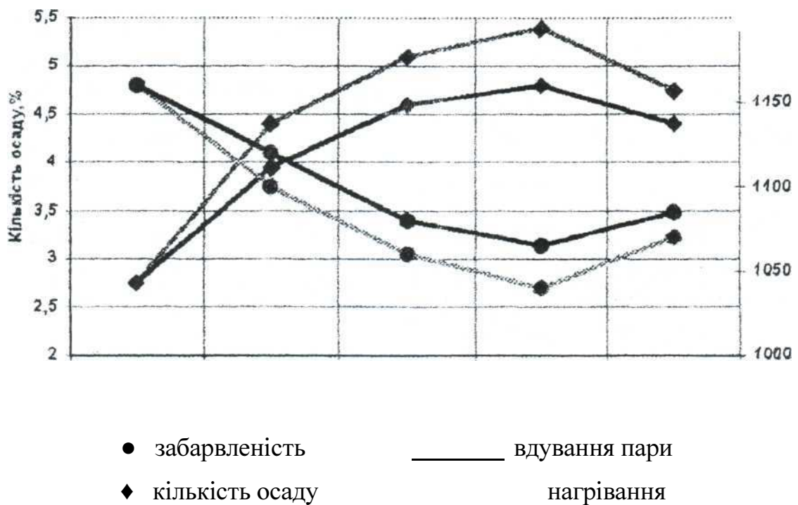
Рис.1. Вплив температури соку на кількість видаленого осаду та величину забарвленості
