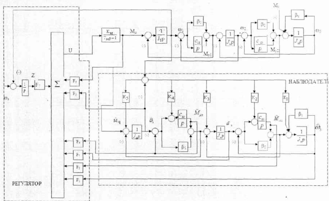
Рис.3. Схема системы оптимального управления главным приводом широкополосного стана горячей прокатки
