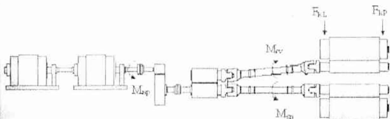
Рис. 2. Схема главного привода клетки кварто широкополосного стана горячей прокатки с шестеренчатой клетью
