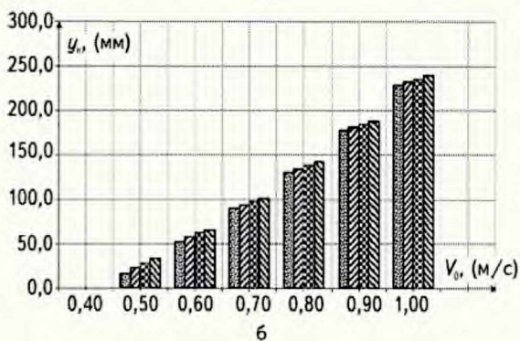
Рис. 3. Зміна значення раціонального розташування зважувальної місткості від швидкості переміщення продукції а) вібраційним, б) стрічковим живильником при різних їх розташуваннях відносно горизонту:
