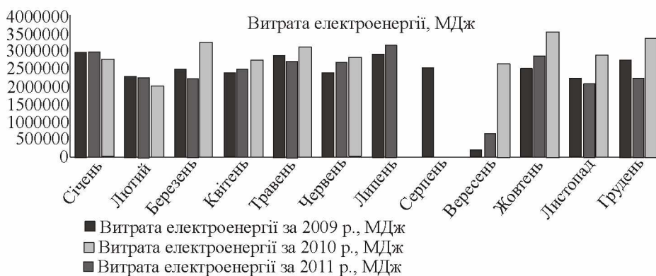
Рис 1. Витрати електроенергії ВАТ «Вінницький олісжиркомбінат»
