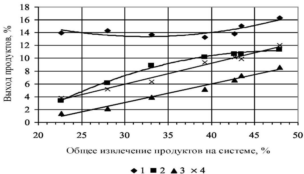
Рисунок 4- Выход промежуточных продуктов измельчения III драной системы мелкой в зависимости от общего извлечения на системе: 1 - средняя крупка; 2 - мелкая крупка; 3 - дунсты; 4 - мука.
