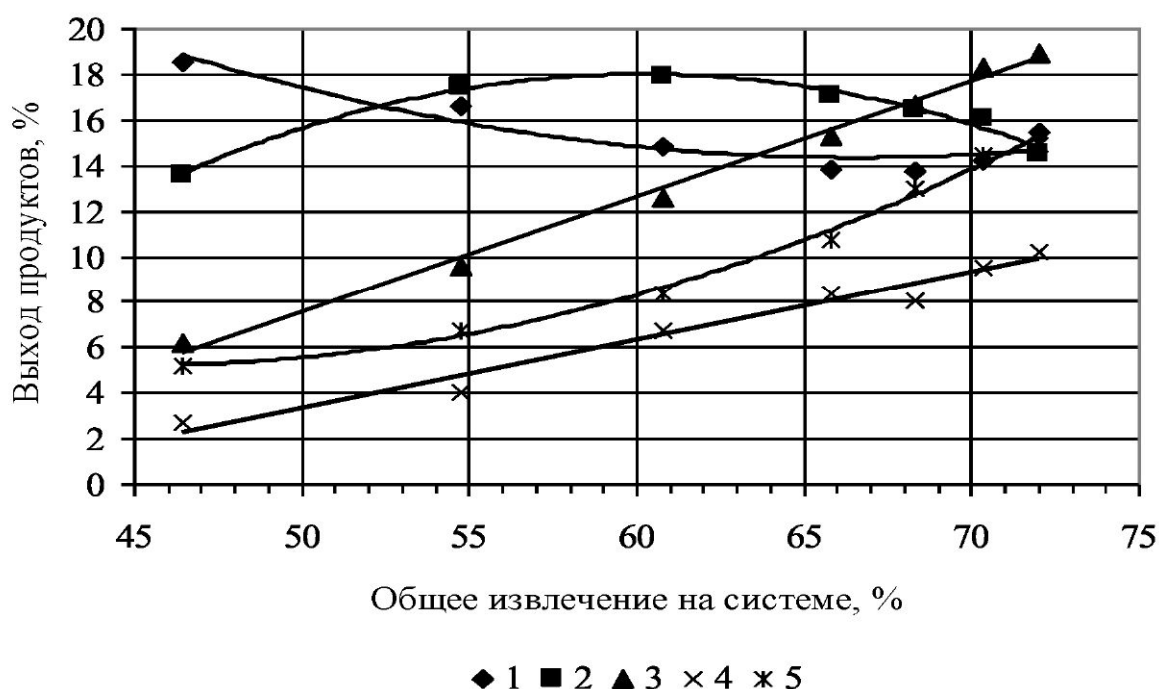
Рисунок 2- Выход круподунстовых продуктов на II драной системе: 1 - крупная крупка; 2 - средняя крупка; 3 - мелкая крупка; 4 - дунсты; 5 - мука.
