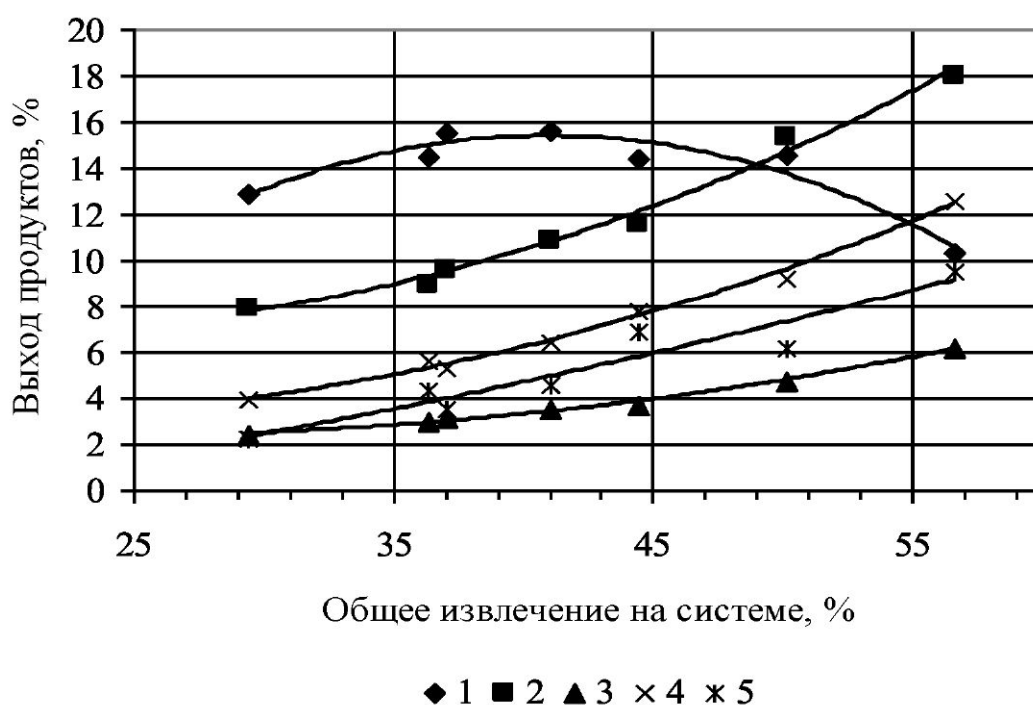
Рисунок 1- Выход круподуновых продуктов при измельчении зерна пшеницы на I драной системе: 1 - крупная крупка; 2 - средняя крупка; 3 - мелкая крупка; 4 - дунсты; 5 - мука.
