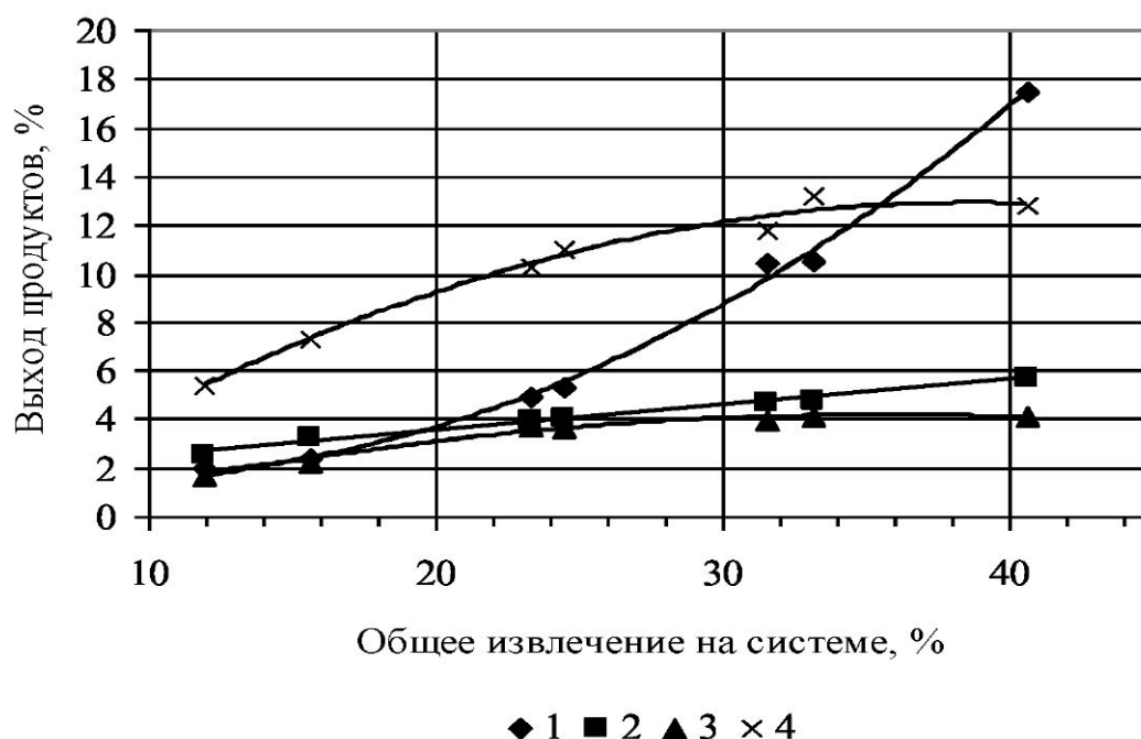
Рисунок 3- Выход промежуточных продуктов измельчения III драной системы крупной в зависимости от общего извлечения на системе: 1 - средняя крупка; 2 - мелкая крупка; 3 - дунсты; 4 - мука.
