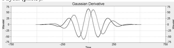
Рис.3. Вейвлет-функція Гауса
