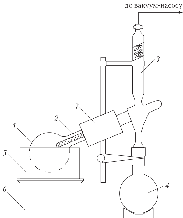
Рис. 2. Апаратурне оформлення мікроработорної установки, працюючої у режимі концентрування та адсорбції ароматичних речовин: 1 – випарювальна колба роторного випарника; 2 – адсорбційна мікроколонка-концентратор; 3 – холодильник; 4 – приймач дистиляту; 5 – станина з нагрівальним елементом; 6 – пристрій живлення роторного випарника; 7 – привід роторного випарника
