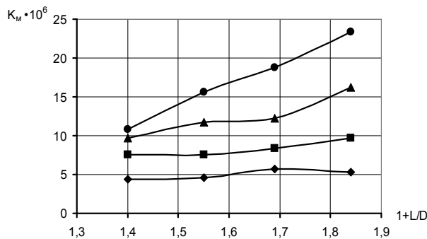
Рис. 2. Залежність загального коефіцієнта розчинення від відносного віддалення точки розміщення зразку \left(1 + \frac{L}{D}\right) при різних частотах коливань вібротранспортувальної системи: ◆ – f = 2 \text{ Гц} , ■ – f = 3 \text{ Гц} , ▲ – f = 4 \text{ Гц} , ● – f = 5 \text{ Гц}
