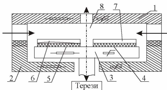
Рис. 2. Принципова схема ДМКВ-1: 1, 2 — верхній і нижній термостатовані блоки; 3 — калориметрична платформа з основним електронагрівником; 4, 5 — перетворювачі теплового потоку; 6 — комірка з пробю дослідного матеріалу; 7 — комірка з еталоном; 8 — робоча камера
