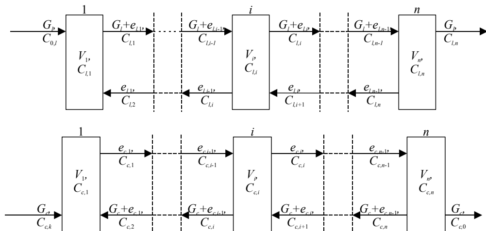
Рис. 3. Параметрична схема комірчастої моделі із зворотними потоками: 0 \leq \tau \leq T — поточний час перебування індикатора рідкої фази в комірці, с; V_i — об'єм i -ої комірки, \text{м}^3 ; C_{li} , C_{ci} — концентрація індикатора в рідкій і твердій фазі, \text{кг}/\text{м}^3 ; e_{li} , e_{ci} — об'ємна швидкість зворотного потоку із (i+1) комірки в i -у та із i -ої в (i+1) -у комірки, \text{м}^3/\text{с}
