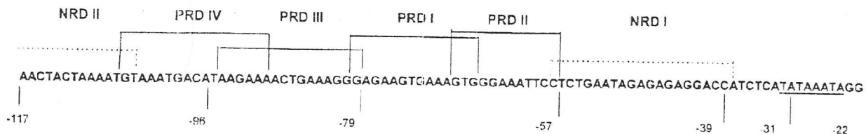
Рис. 1. Організація регуляторних послідовностей гена ІФН-В людини. Цифрами вказано відстань у нуклеотидах від початкової точки зчитування. Відмічено TATAA-бокс (TATA), позитивні регуляторні домени (PRD) і негативні регуляторні домени (NRD)
