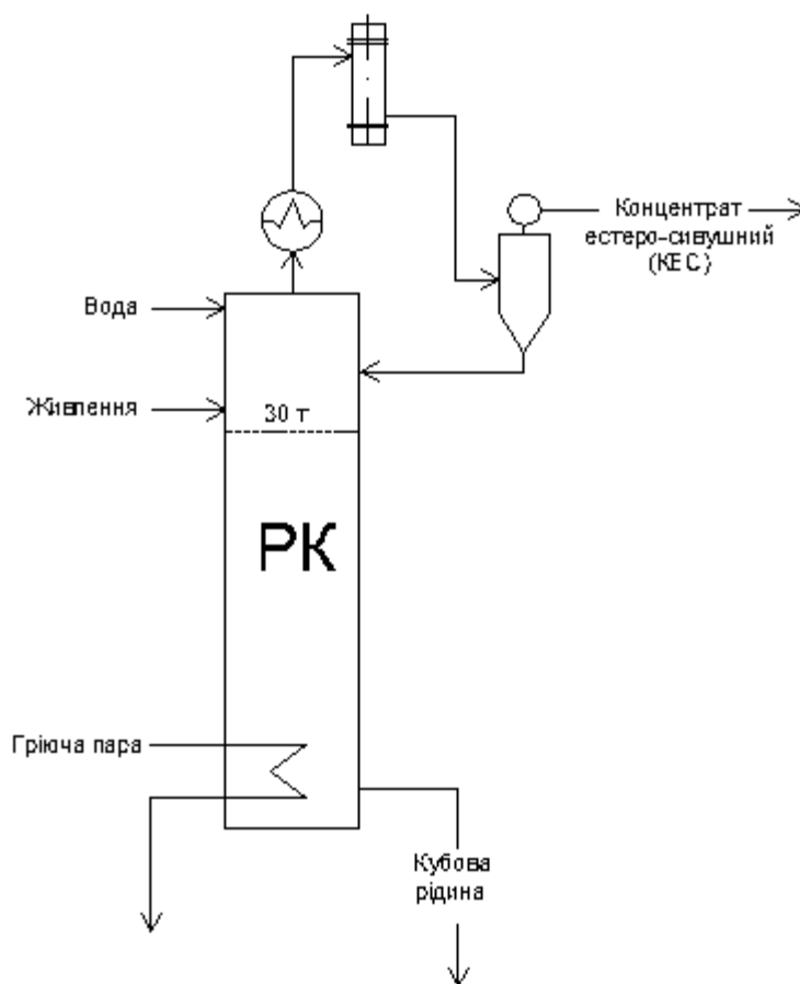
Рис.1. Схема роботи РК
