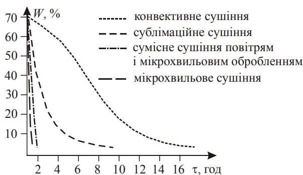
Рис. 1. Принциповий графік залежності зміни вологовмісту W харчових продуктів під час сушіння мікрохвильовим і конвективним способами у різних комбінаціях
