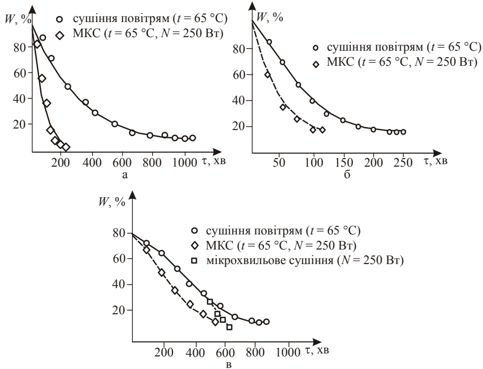
Рис. 2. Графік залежності зміни вологовмісту W під час сушіння мікрохвильовим і конвективним способами у різних комбінаціях: а — яблуку; б — моркви; в — слив
