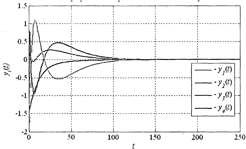
Рисунок 3 – Графіки перехідних процесів спостережень станів системи y(t)
