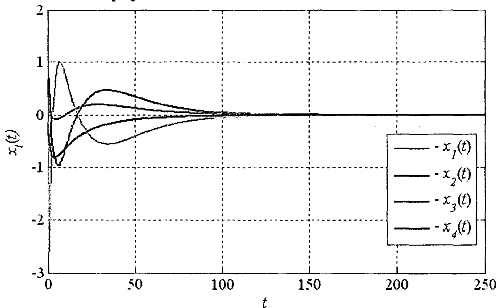
Рисунок 4 – Графіки перехідних процесів оптимальних оцінок станів системи x(t)
