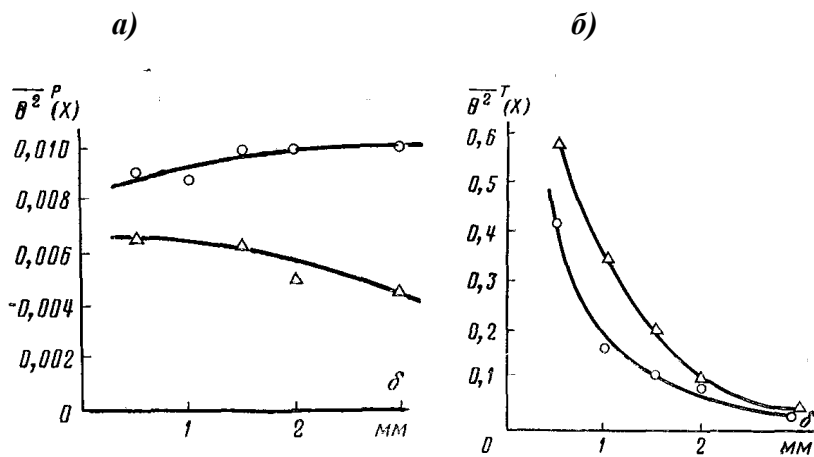
Рис.10. Зміни \overline{\theta^2}^P (а) і \overline{\theta^2}^T (б) в залежності від відстані до гріючої стінки при тепловому потоці: \Delta – 197300 і \circ – 257300 Вт/м 2
