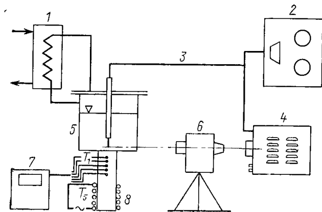
Рис.2. Дослідна установка для вимірювання пульсацій температури: 1 – конденсатор; 2 – магнітофон; 3 – мікро термопара; 4 – осцилограф; 5 – дослідна посудина; 6 – кінокамера; 7 – самогрівець; 8 – електронагрівач
