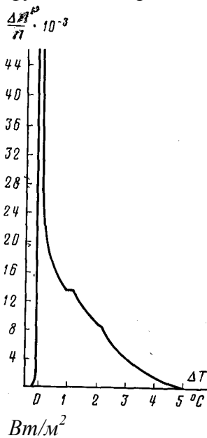
Рис.5. Розподіл щільності ймовірності пульсацій температури на відстані від стінки 0,5 мм при тепловому потоці 257300 \text{ Вт/м}^2
