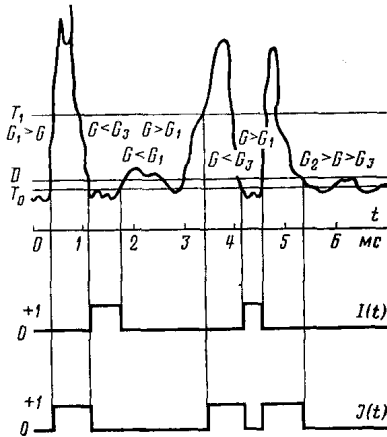
←Рис.3. Сигнал мікро термопару і відповідна йому функція переміжності
