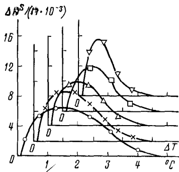
Рис.7. Розподіл щільності ймовірності пульсацій температури в перегрітому рідкому шарі
