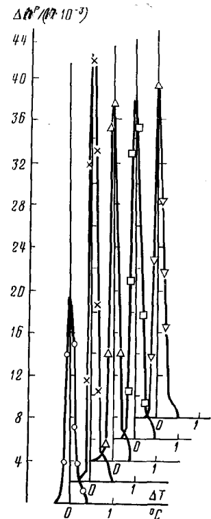
Рис.5. Розподіл щільності ймовірності пульсацій температури на відстані від стінки 0,5 мм при тепловому потоці 257300 \text{ Вт/м}^2
