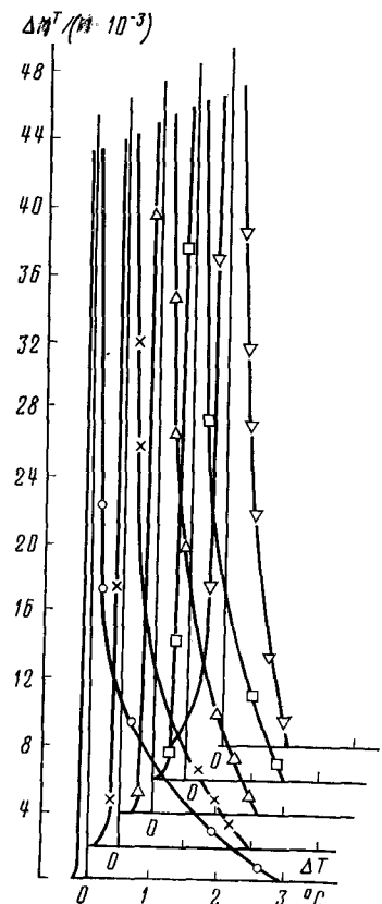
Рис.9. Розподіл щільності ймовірності пульсацій температури в області рідини на різній відстані від гріючої стінки
