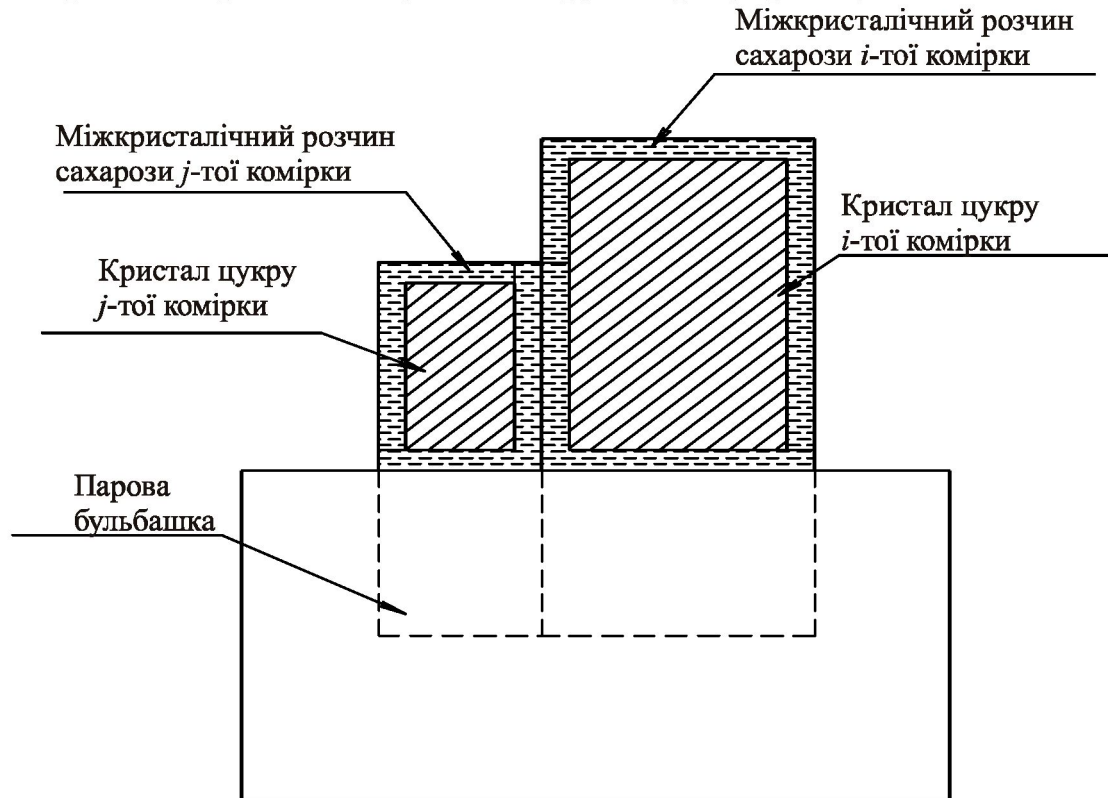
Рис. 2. Двовимірна модель міжкристалічний розчин меншої j -ої комірки—кристал меншої j -ої комірки сахарози—парова бульбашка—кристал більшої i -ої комірки сахарози—міжкристалічний розчин більшої i -ої комірки при масовій кристалізації утфелю
