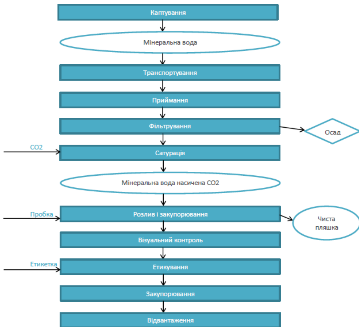
Рис.1.4. Технологічна схема виробництва ТОВ «Тальнівський завод «Мінводи»
