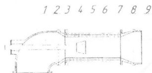
Рис. 3. ГКА (кавітаційний змішувач) зі змінною проточною робочою камерою з керамічного матеріалу
