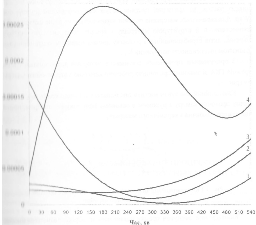
Рис. 2. Кінетичні залежності швидкості ґношування зразків, \Delta V / \Delta t (1, 2, 3, 4 – номери зразків за таблицею).
