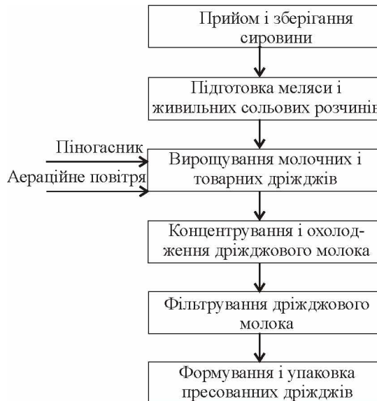
Рис. 1. Схема виробництва пресованих дріжджів
