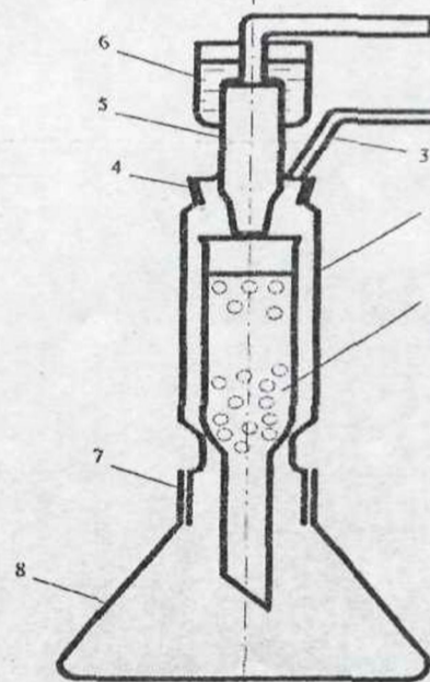
Рис.1. Схема лабораторної установки для адсорбційного очищення сортівки : 1 – колонка з адсорбентом; 2 – вакуумна сміть; 3 – вакуум-відвід; 4, 7 – шліф; 5 – шліф-кран; 6 – сміть живлення; 8 – сміть для очищеного розчину.
