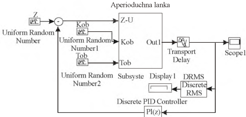
Рис. 2. Схема моделювання САР з ПІ регулятором
