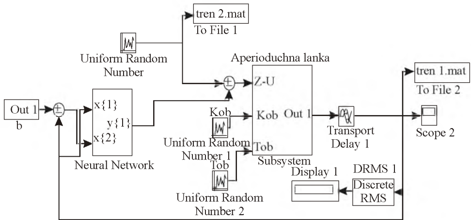
Рис. 8. Схема моделювання САР з HMP на етапі побудови НІ
