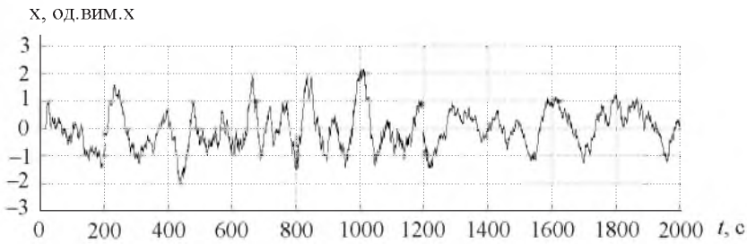
Рис. 12. Графік процесу регулювання САР з ПІ-регулятором при k_{ob} \rightarrow \text{const} , T_{ob} \rightarrow \text{var}
