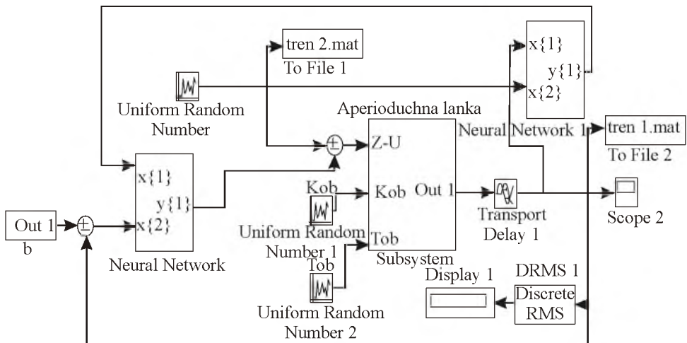
Рис. 9. Схема моделювання САР з HMP і НІ на другому етапі
