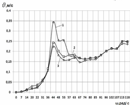
Рис. 3. Залежність віброшвидкості від кутової частоти приводного валу
