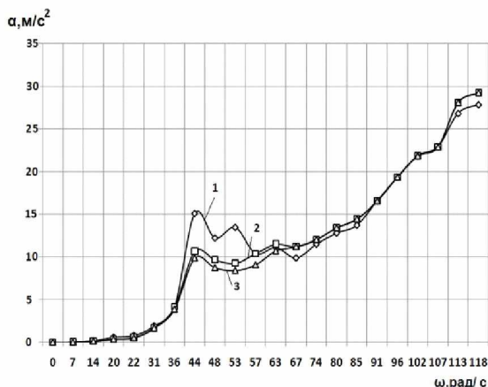
Рис. 4. Залежність віброприскорення від кутової частоти приводного валу
