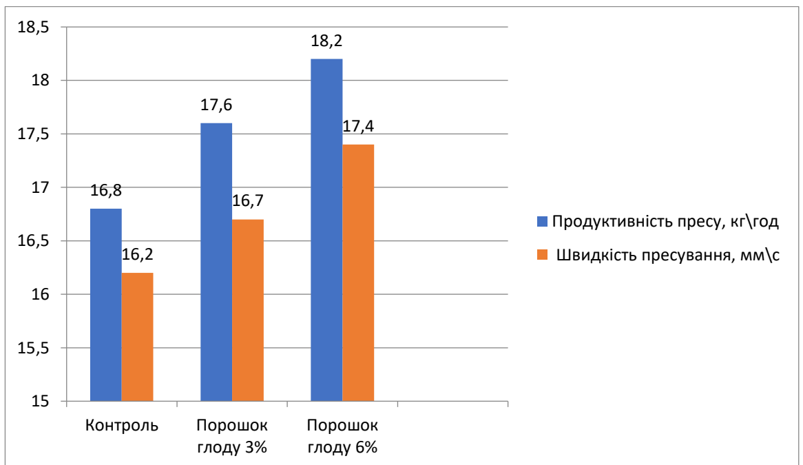
Рис. 2. Вплив порошку глуду на параметри пресування макаронних виробів
