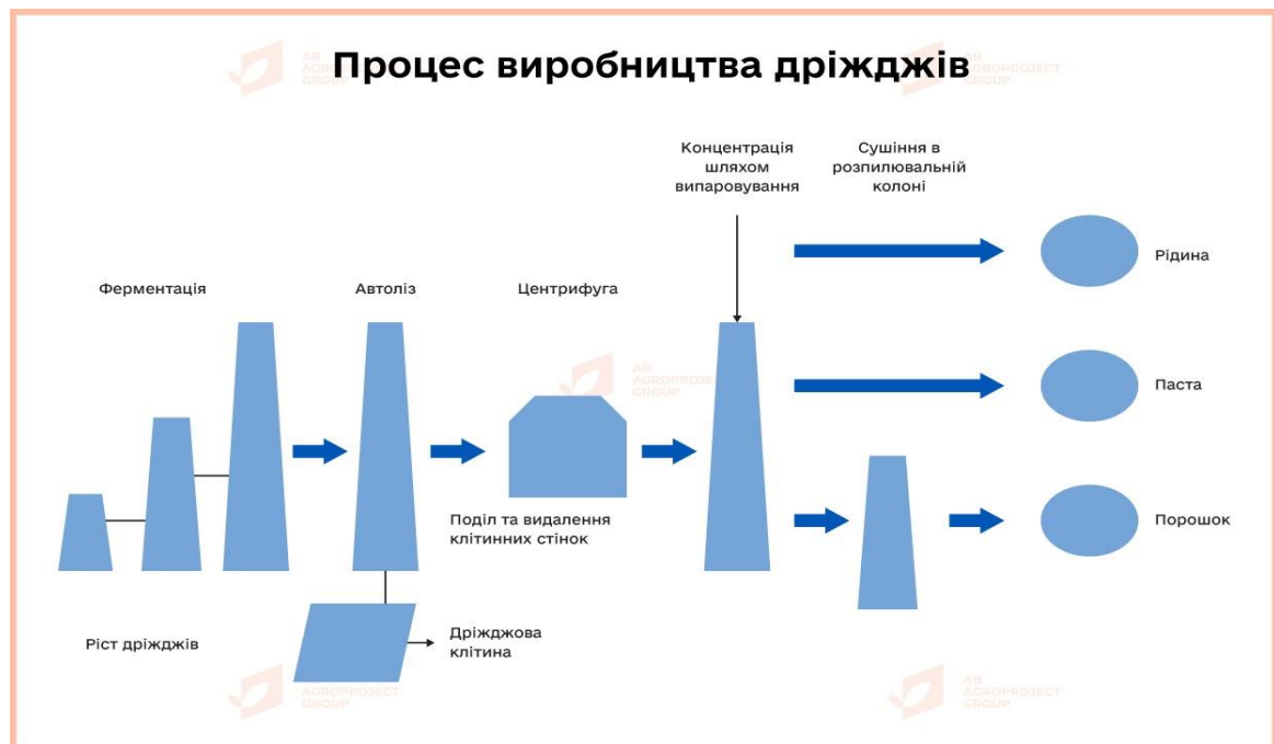
Рис. 3.6. Процес виробництва сухих порошкових дріжджів на ТОВ «Компанія Ензим» як основного інгредієнта для виробництва «Львівські дріжджі без глютену - Gluten Free»
