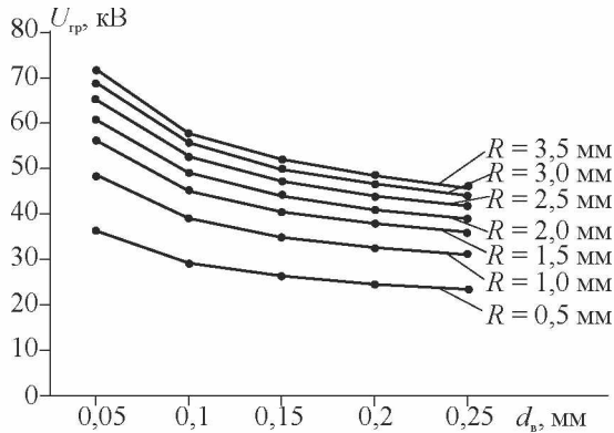
Рис. 7. Графік залежності граничних значень напруги на ізоляторі U_{\text{гр}} , при яких відбувається пробій включення (пори), залежно від діаметра пори d_{\text{в}} для різних значень радіуса заокруглення R кінцевої частини стрижня
