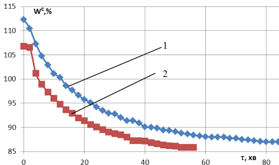
Рис.1. Криві комбінованого сушіння пасти рисового борошна з буряковим барвником при співвідношенні: 1 – 1:0,75, 2 – 1:1.
