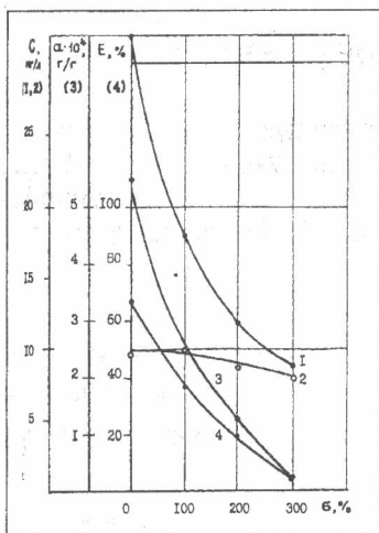
Рис.4 Зміна початкової (1), кінцевої (2) концентрації барвника, питомої адсорбції (3) і ефекту знебарвлення (4) при різних кратностях розбавлення
