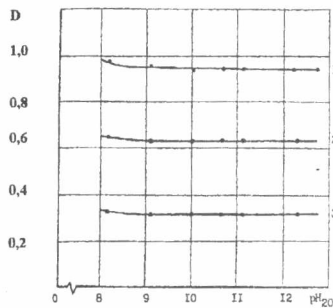
Рис. 2 Залежність оптичної густини розчину кислотного червоного 2С від pH_{20} при концентрації, мг/л: 1 - 32,3; 2 - 21,5 3; 3 - 10,8
