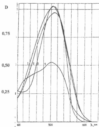
Рис. 3 Спектри кислотних барвників: 1 - червоного 2С при pH 12,25; 2 - червоного 2С при pH 8,75; 3 - ясно-червоного при pH 8,75; 4 - ясно-червоного при pH 12,25;
