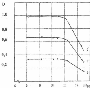
Рис. 1 Залежність оптичної густини розчину кислотного ясно-червоного від pH_{20} при концентрації, мг/л: 1 - 32; 2 - 21,3; 3 - 10,6
