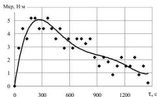
Рисунок 2 - Влияние продолжительности замеса на смену крутящего момента, при \omega = 0,8 \text{ с}^{-1}
