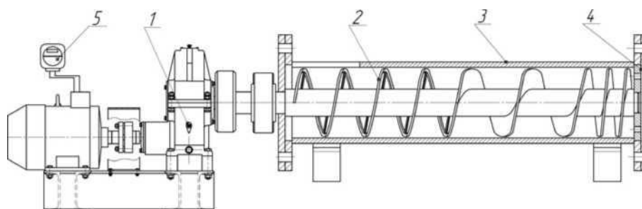
Рисунок 1 - Экспериментальная установка непрерывного действия для замеса теста: 1 - привод; 2 - рабочий орган (шнеки); 3 - корпус; 4 - стабилизирующая решетка; 5 - прибор "УОБТСЯАНТ" для измерения электрической мощности.
