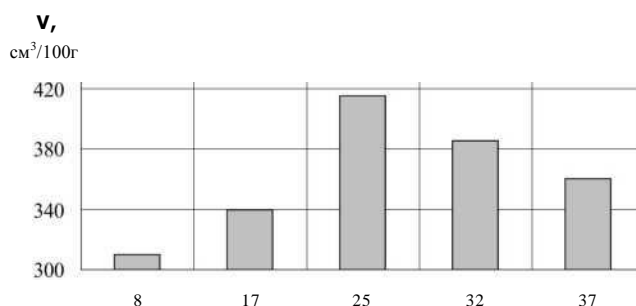
Рисунок 3 - Суммарное выделение диоксида углерода за 3 часа, брожения теста при различной удельной работе Ауд, Дж/г.
