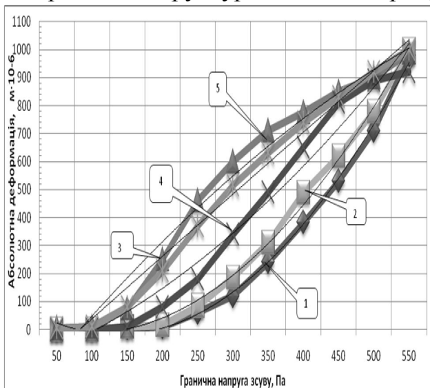
Рисунок 7 - Залежність абсолютної деформації паштетів від напруги зсуву
