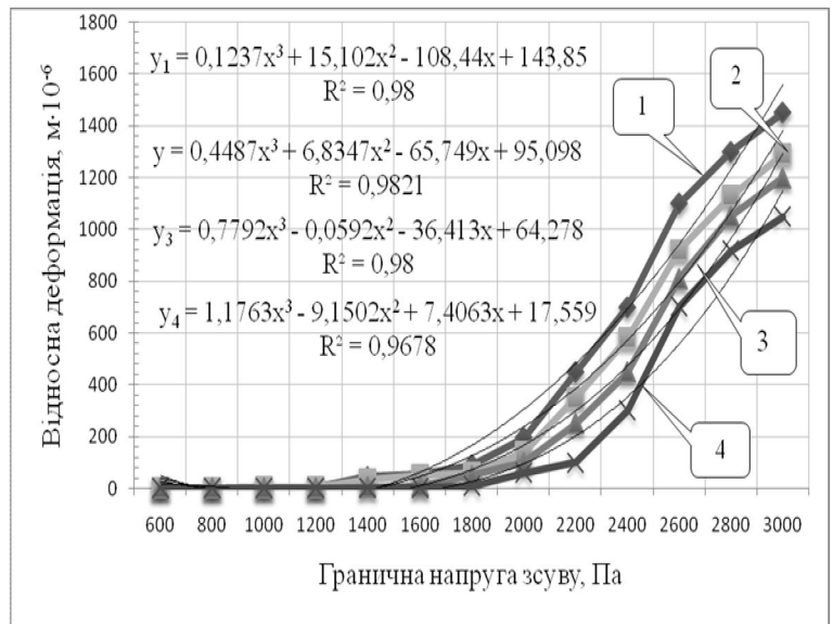
Зразки: 1 – гелю альгінату кальцію; 2 – 1:4 ГПН: гелю альгінату кальцію; 3 – 1:9 ГПН: гелю альгінату кальцію; 4 – 1:14 ГПН: гелю альгінату кальцію
