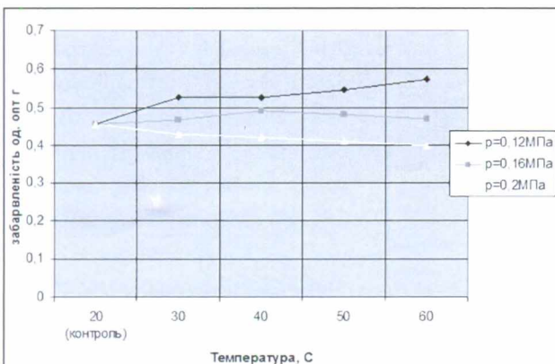
Рис. 3. Залежність зміни показника забарвленості від температури
