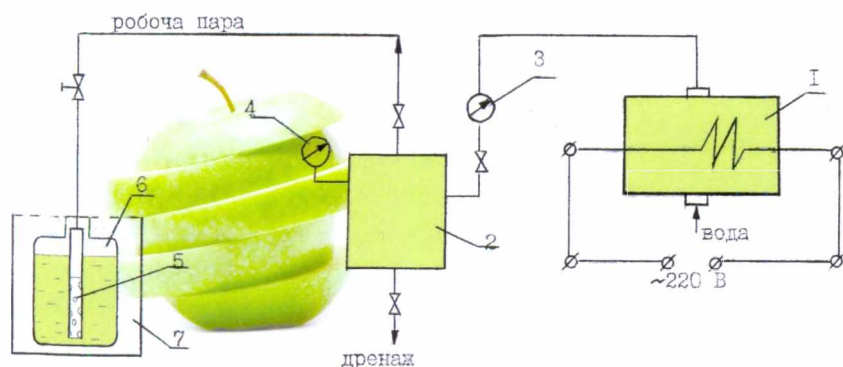
Рис. 1. Схема лабораторної установки:
