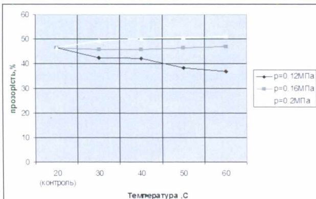
Рис. 4. Залежність зміни показника прозорості від температури
