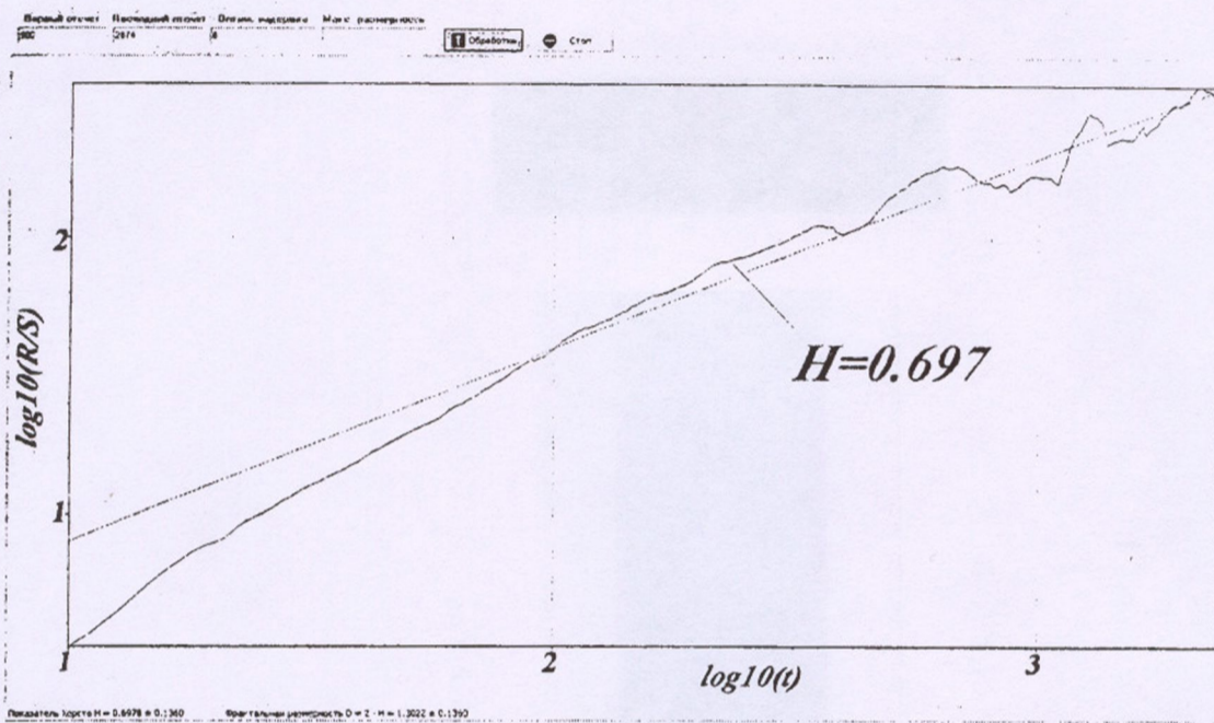
Рис. 6. Розрахунок показника Херста для витрати бурякової стружки
