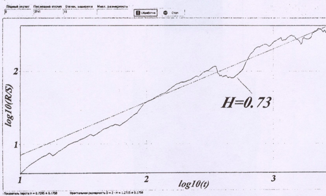
Рис. 7. Розрахунок показника Херста для витрати дифузійного соку
