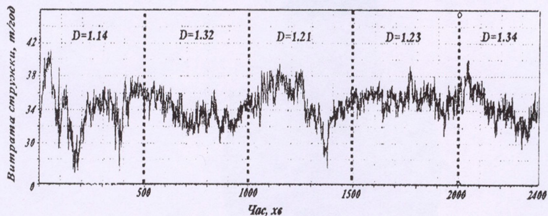
Рис.2. Визначення фрактальної розмірності зміни витрати бурякової стружки.
