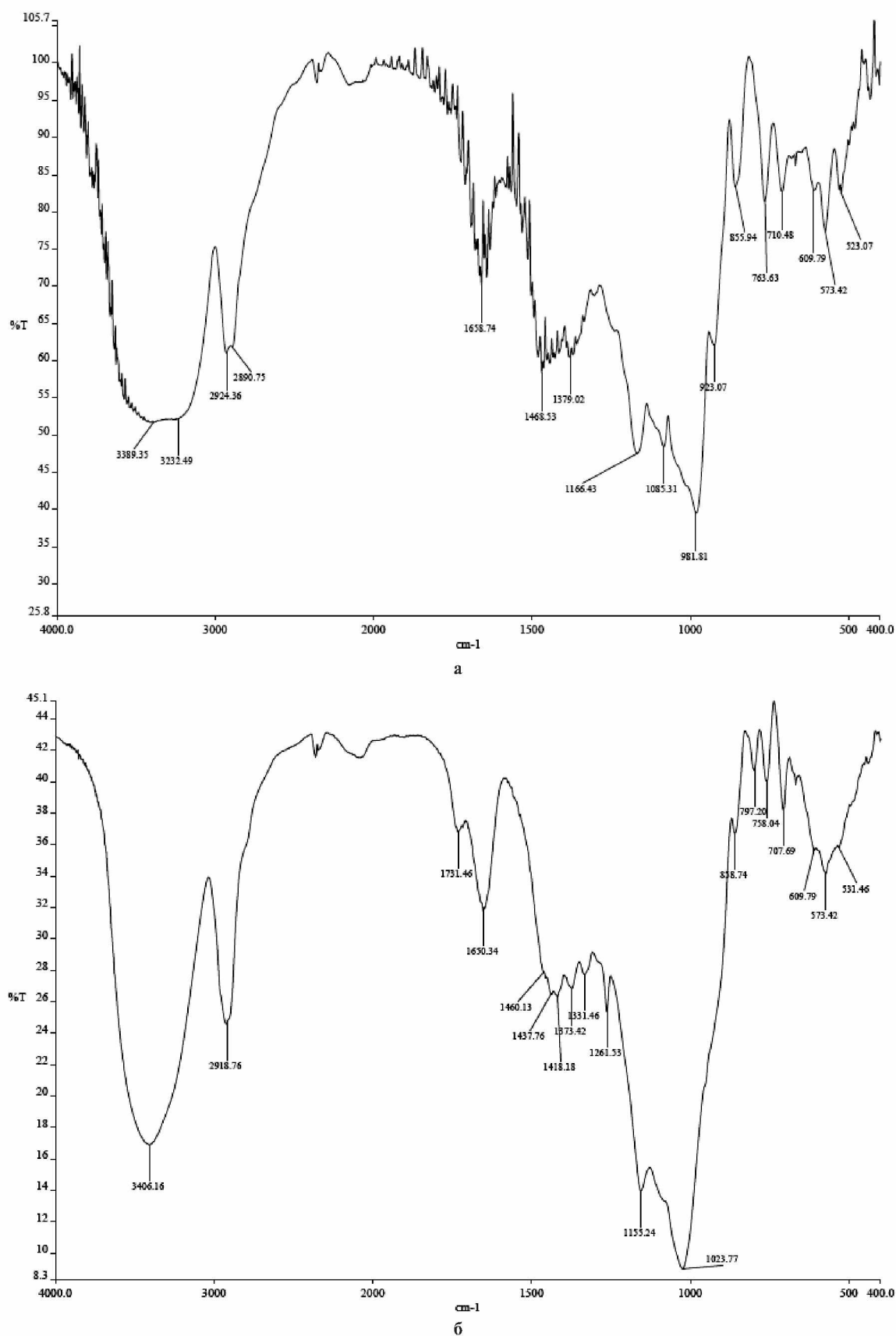
Рис. 1. ІЧ-спектри вихідного нативного картопляного крохмалю (а) та його естерифікованого похідного (б)
