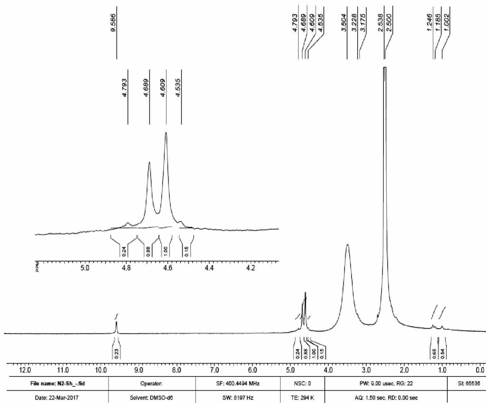
Рис. 2. ЯМР-спектри вихідного нативного картопляного крохмалю (а) та його стерифікованого похідного (б)
