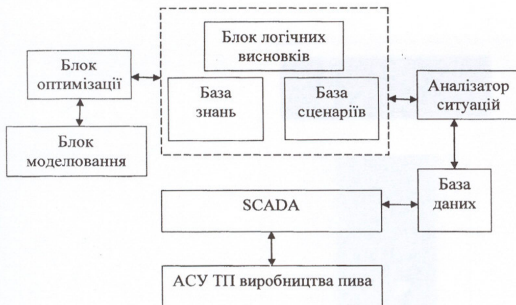
Рис. 2. Структура системи автоматизації виробництва пива
