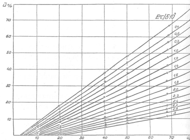
Рис.2. Узагальнені криві терморадіаційного сушіння картопляного крохмалю
