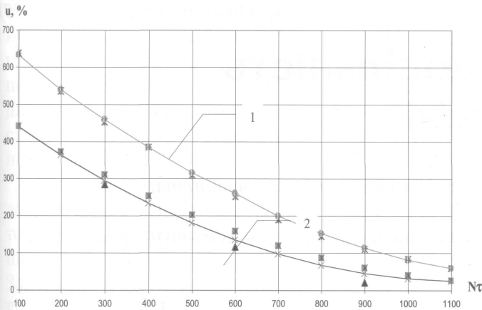
Рис. 3. Залежність вологовмісту жому від комплексної величини N\tau
