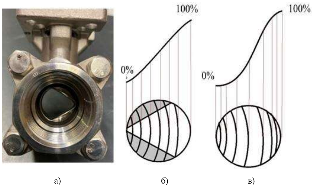
Рис. 6. Запірно-регулювальний пристрій стабілізуючого контура РОУ: а) кульовий кран; б), в) порівняльні характеристики зміни витрат води в стабілізуючому контурі РОУ при використанні кульового крана з V-подібним вирізом під кутом 60^\circ і звичайного кульового крана
