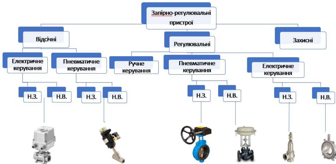
Рис. 1. Узагальнена класифікація промислових запірно-регулювальних пристроїв цукрового виробництва:
