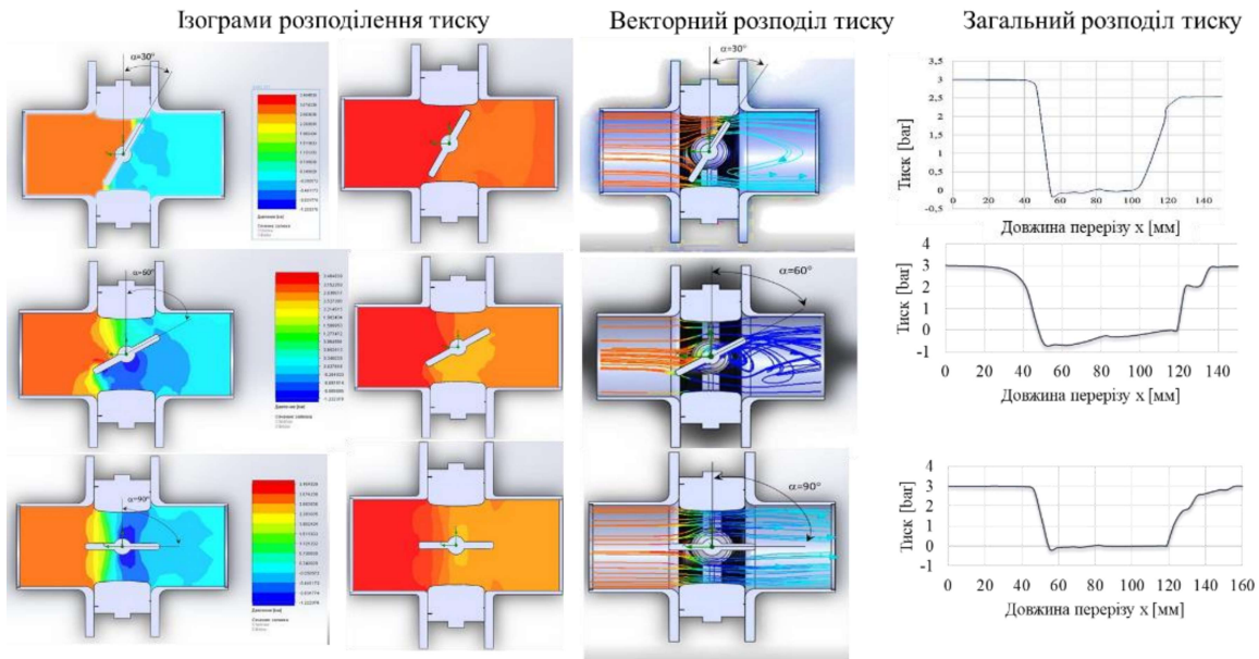
Рис. 3. Моделі, побудовані для отримання графічних залежностей розподілення тисків, для встановленого кута відкриття диска заслінки: 30°, 60°, 90°
