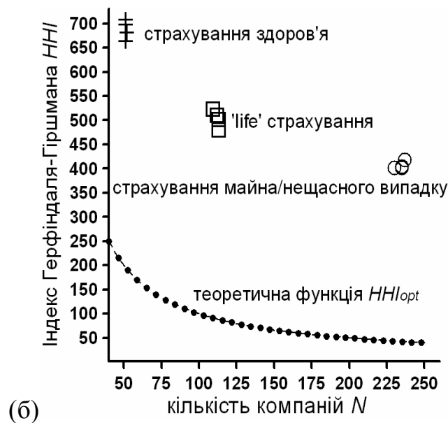
Рисунок 1. Реальні значення індексів Герфіндаля-Гіршмана в 2005–2009 роках: (а-б) теоретична функція HHI_{opt} = 10000/N для рівномірного розподілу страхового ринку Німеччини
