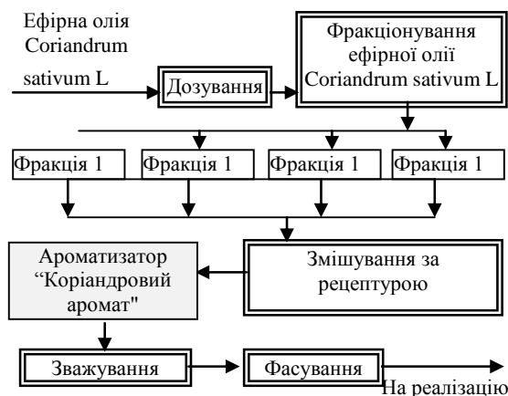
Рис. 1 Схема отримання ароматизатору з коріандрової ефірної олії
